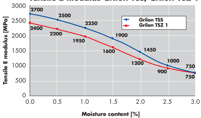
Tensile E modulus Grilon TSS, Grilon TSZ 1
