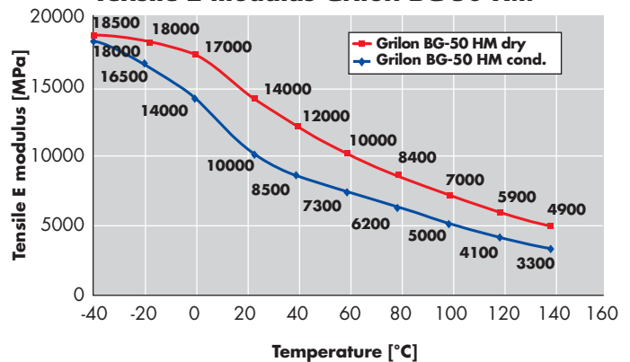
Tensile E modulus Grilon BG-50 HM
