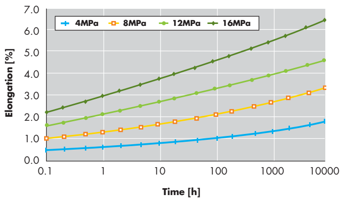
Creep curves Grilon TSG-50/4 at 23°C / 50% r.h.
