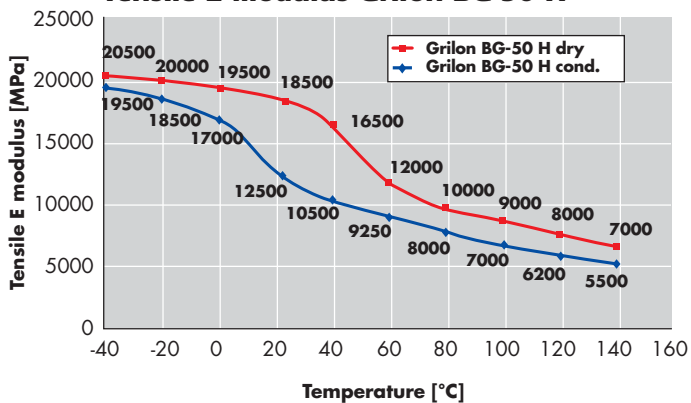
Tensile E modulus Grilon BG-50 H
